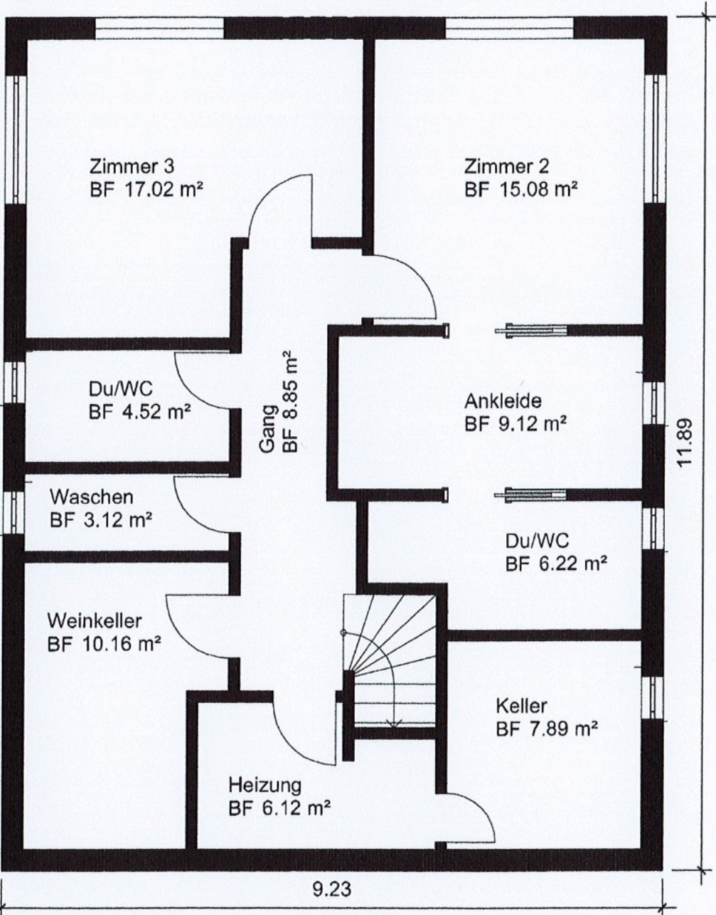
GRUNDRISS ERDGESCHOSS
